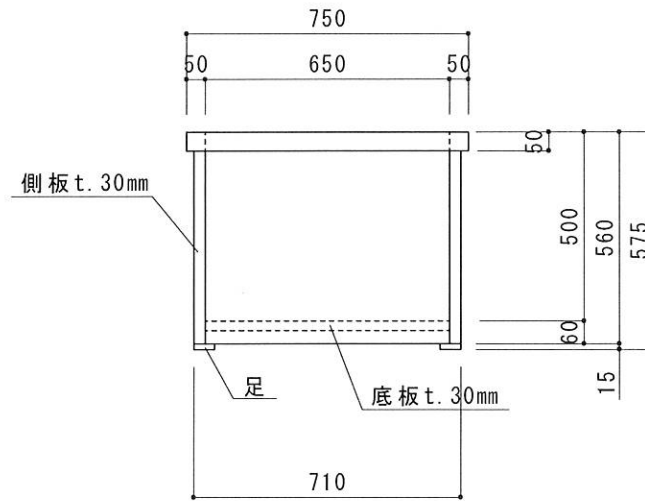
右側面図
