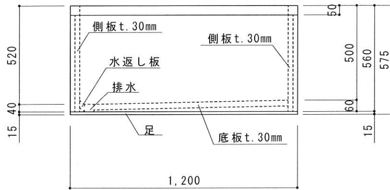
側面図
